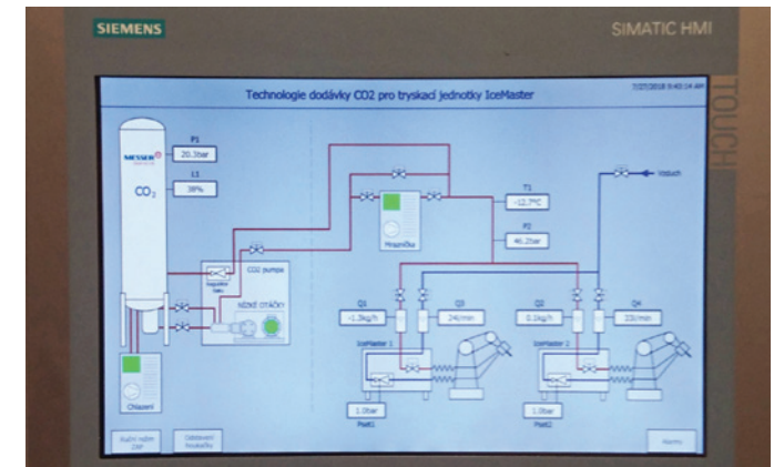
Obr. 4 - PLC – automatizace procesu v reálném čase
