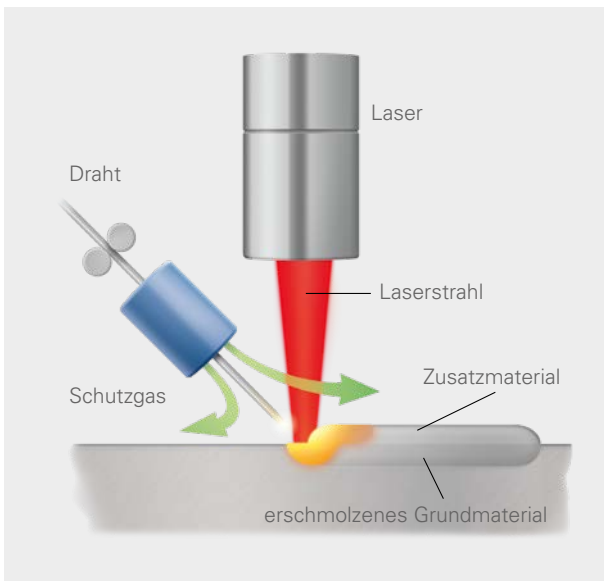
Laserauftragschweißen mit Draht
