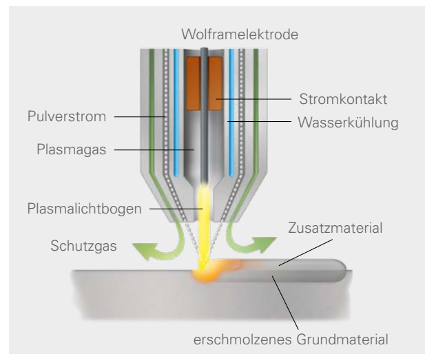
Plasma-Pulver-Auftragschweißen
